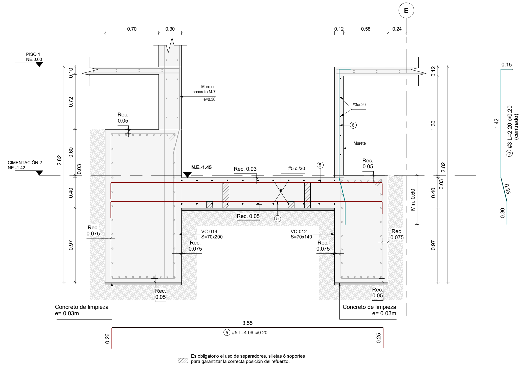
CORTE FS-2 Escala 1 : 25
