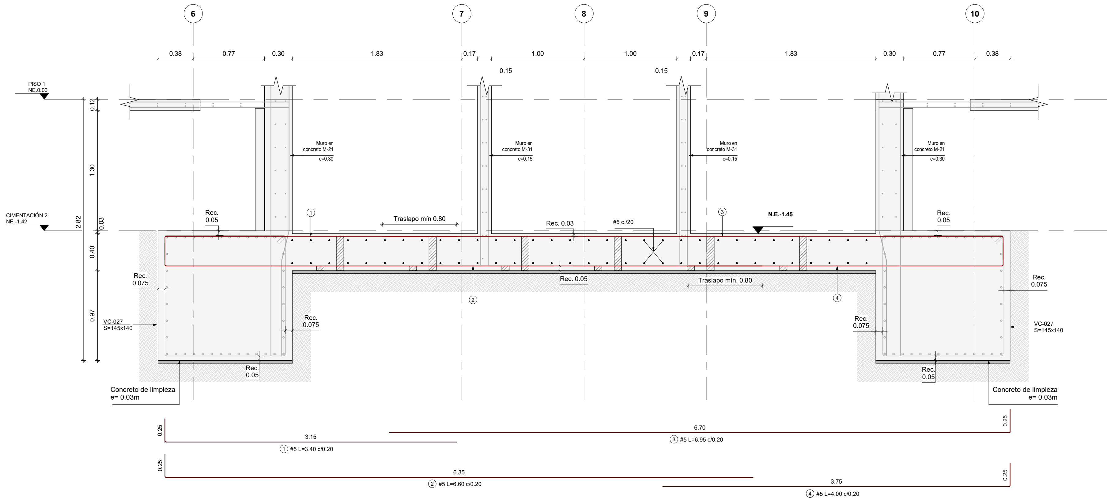
CORTE FS-1 Escala 1 : 25
