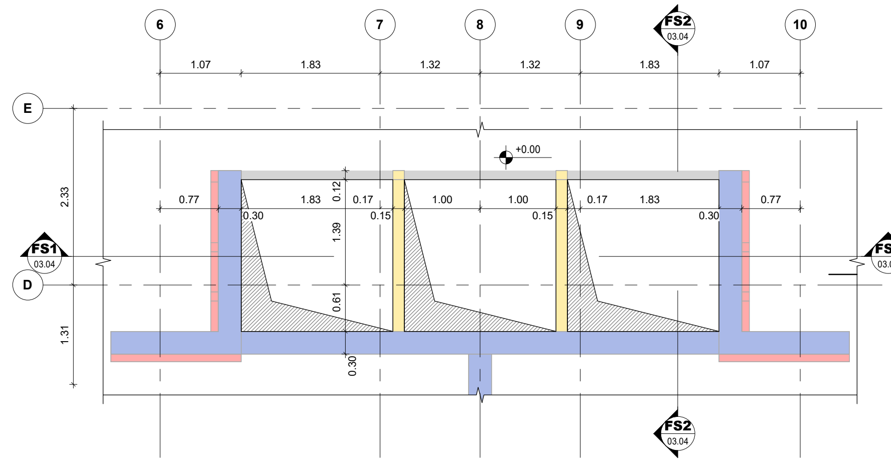
PLANTA FOSO DE ASCENSORES NIVEL 0.00 Escala 1 : 50
