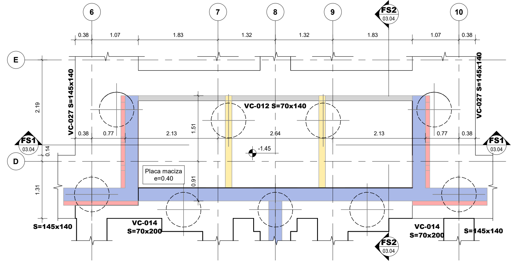
PLANTA DE CIMENTACIÓN FOSO ASCENSORES Escala 1 : 50
